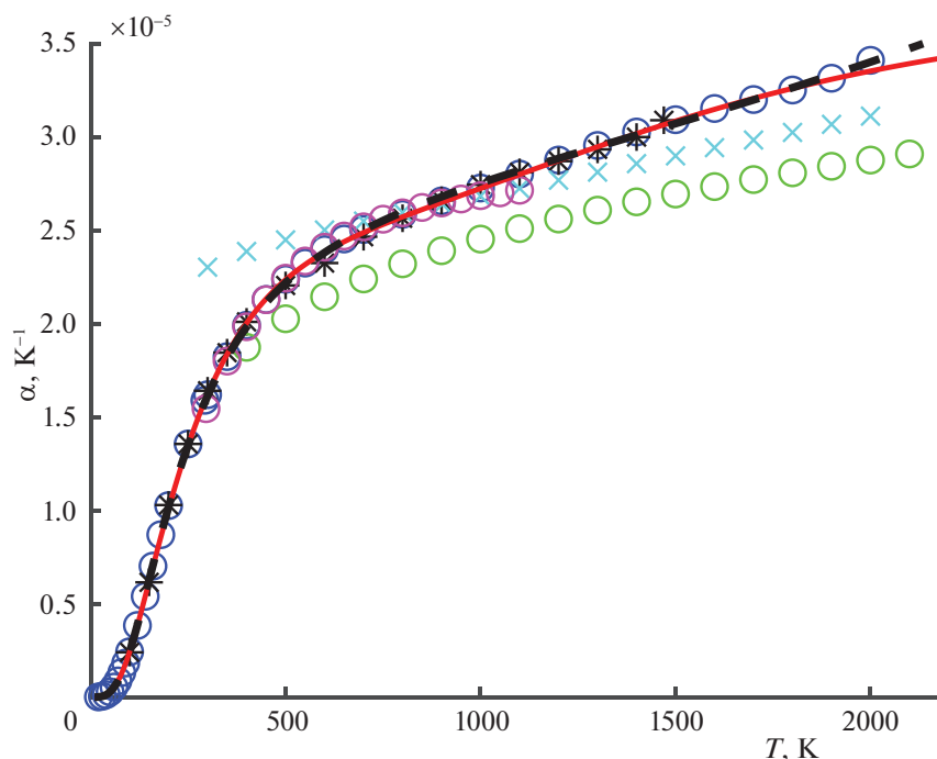
Рис. 2. Зависимости коэффициента термического расширения \alpha - \text{Al}_2\text{O}_3 от температуры, P^\circ = 1 бар. Линии – результаты расчета с использованием C_p -подхода (красная кривая) и C_v -подхода (черная пунктирная кривая). Символами обозначены экспериментальные данные: синие круги [35], черные звездочки [36], розовые круги [37], голубые крестики [34], зеленые круги [33].
