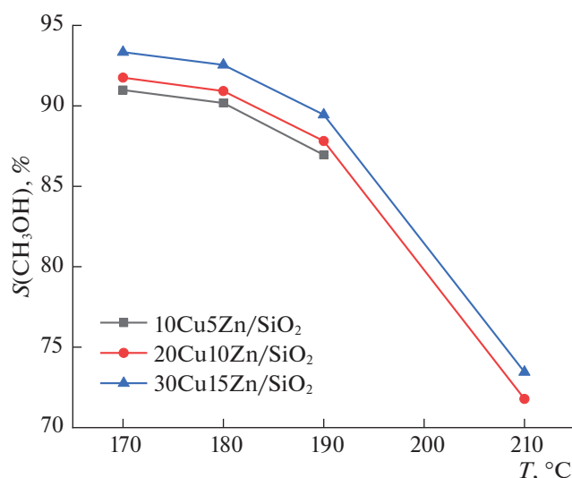
Рис. 5. Зависимости селективности по \text{CH}_3\text{OH} от температуры при P = 20 атм для образцов \text{CuZn/SiO}_2 .
