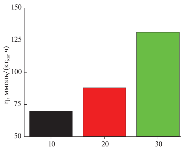
Рис. 4. Зависимость производительности по CH 3 OH ( \eta ) от давления (атм) для образца 10Cu5Zn/Al 2 O 3 при 170°C.
